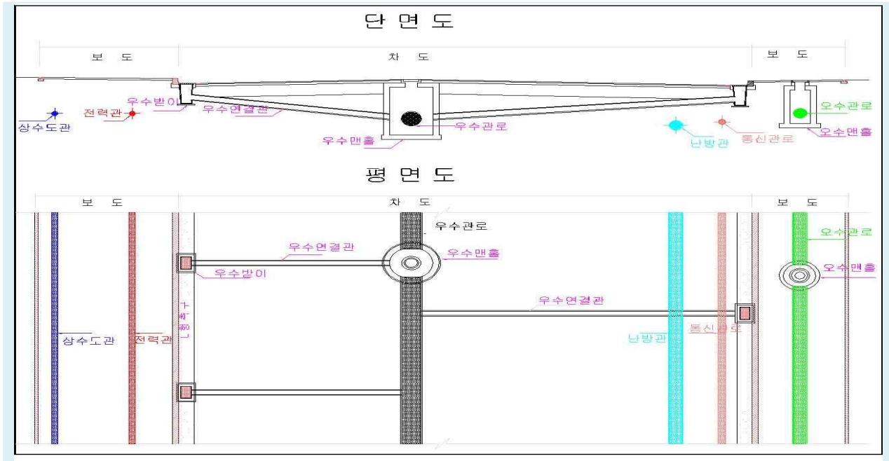
[그림 1] 도로 지하매설물 표준 예시도
